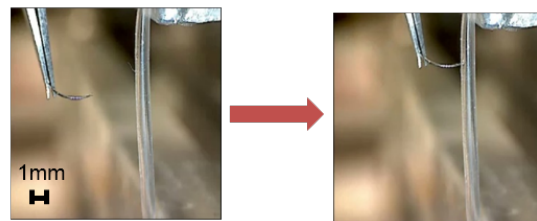
力覚フィードバックによる模擬血管刺入実験の様子 (オペレータが「針が接触した」と感じた瞬間に停止している)
