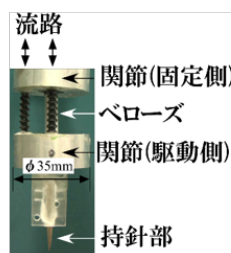
液圧駆動関節
